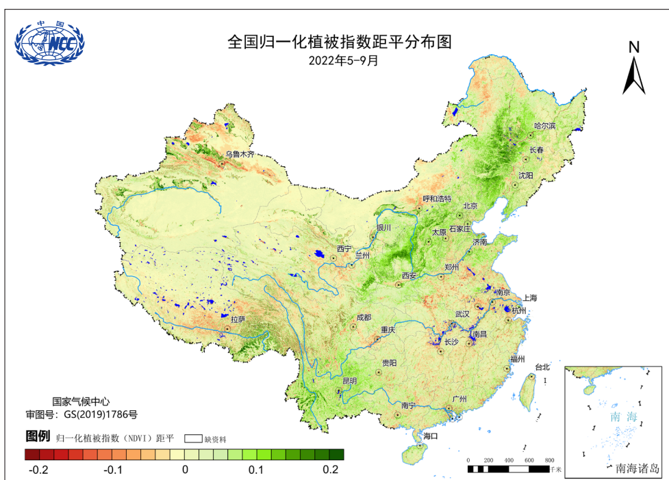
图59 2022年5-9月全国植被指数距平分布
