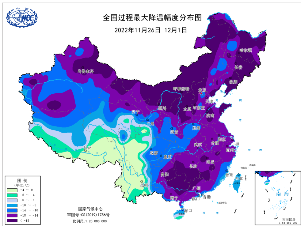
图49 2022年11月26日-12月1日全国过程最大降温幅度分布(单位:℃)
