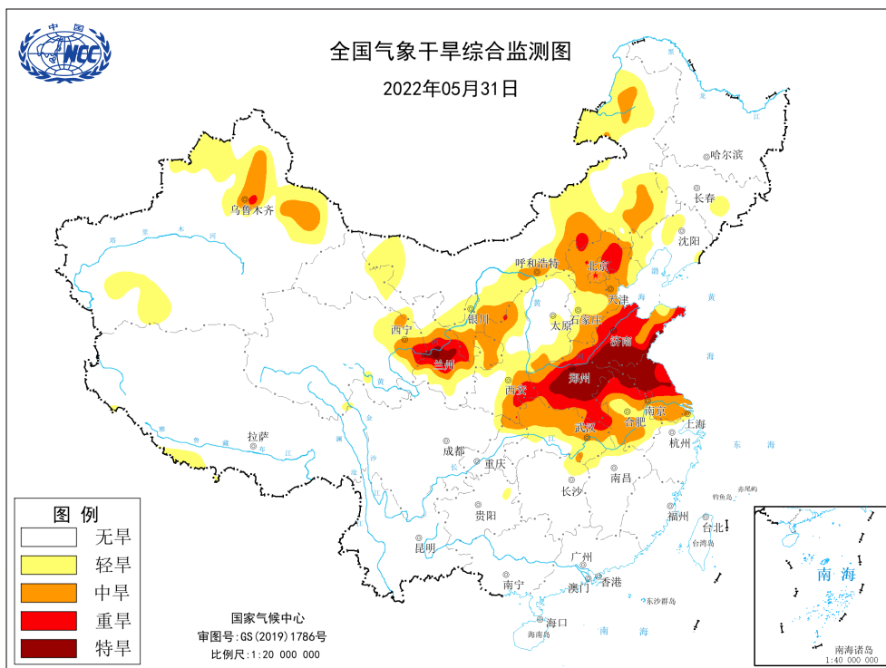
图41 2022年5月31日全国气象干旱综合监测图
