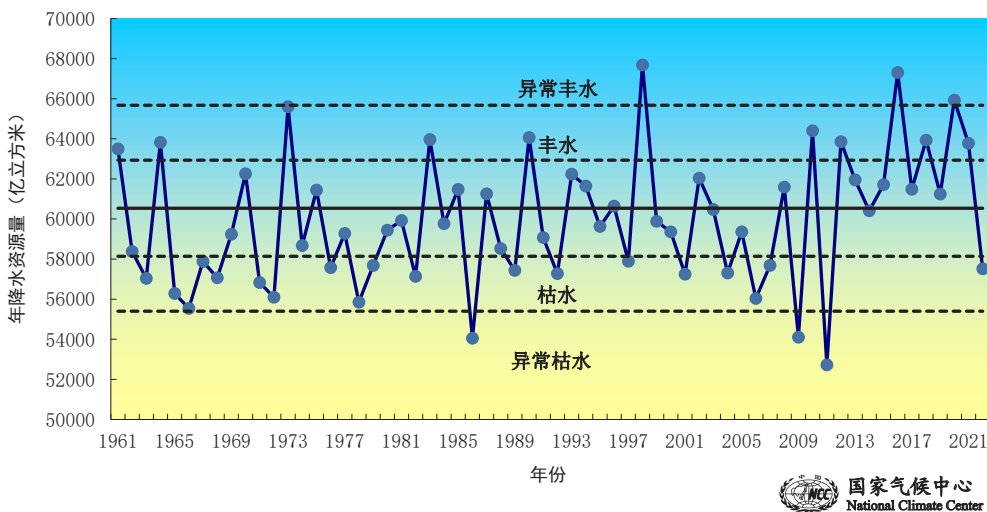
图53 1961-2022年全国年降水资源量变化(单位: 亿立方米)
