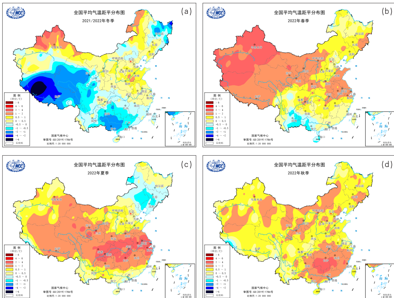
图5 2022年全国四季 (a: 冬; b: 春; c: 夏; d: 秋) 平均气温距平分布 (单位: °C)
