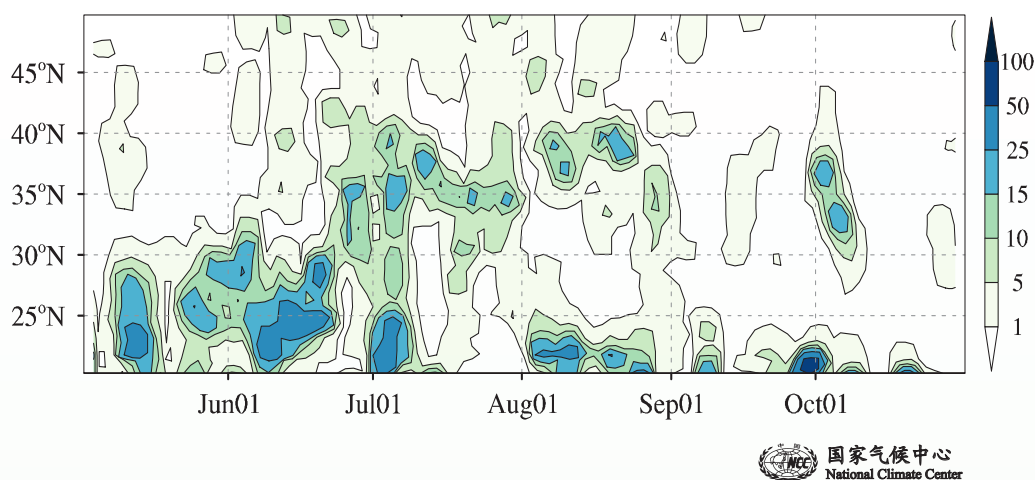
图35 2022年5-10月110°E-120°E平均候降水量纬度-时间剖面 (单位:毫米,图中阴影和等值线为5天滑动平均结果)
