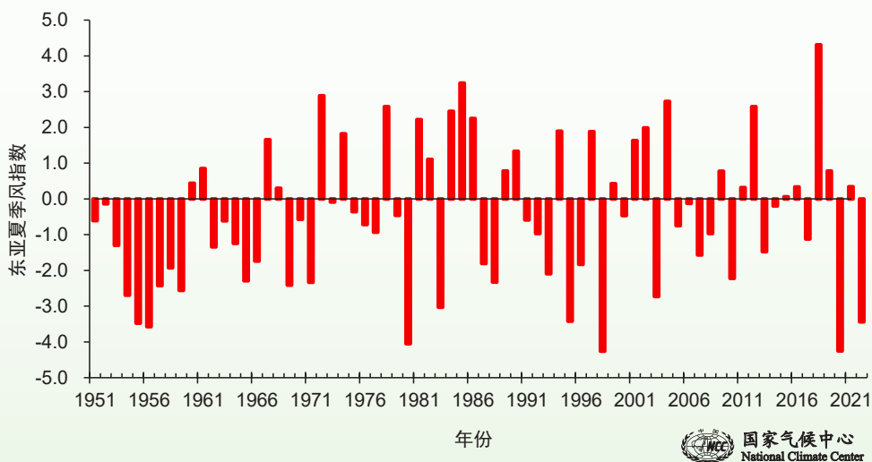
图34 1951-2022年东亚副热带夏季风强度指数历年变化
