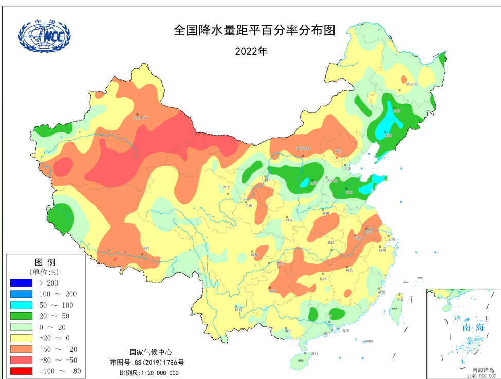
图16 2022年全国降水量距平百分率分布 (单位: %)
