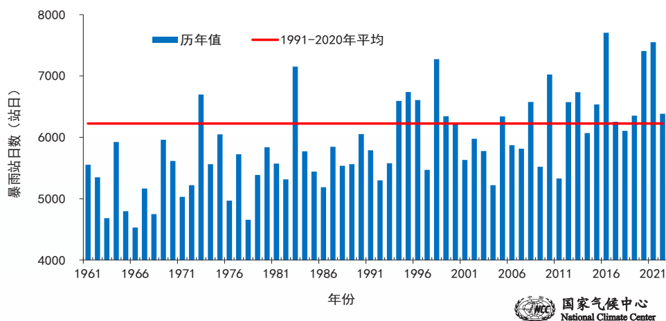
图22 1961-2022年全国暴雨站日数历年变化 (单位: 站日)
