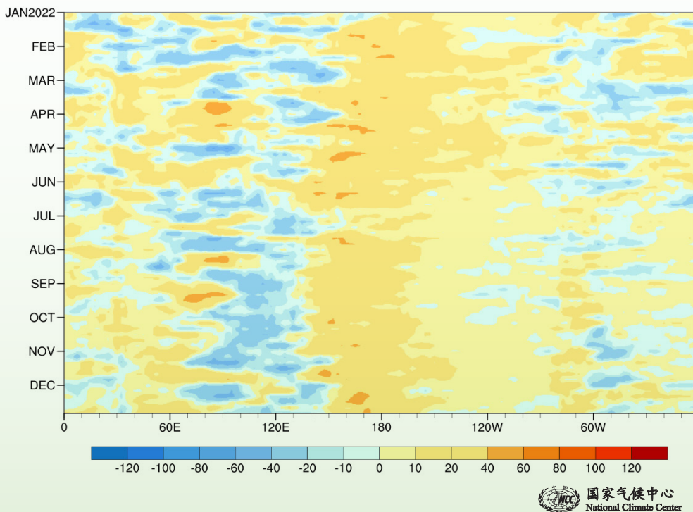
图27 2022年1-12月赤道地区 (5°S~5°N) 射出长波辐射通量距平时间—经度剖面 (单位: 瓦/平方米)
