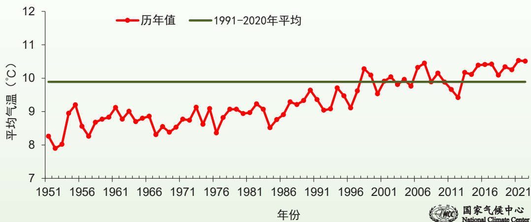
图1 1951-2022年全国平均气温历年变化 (单位: °C)
