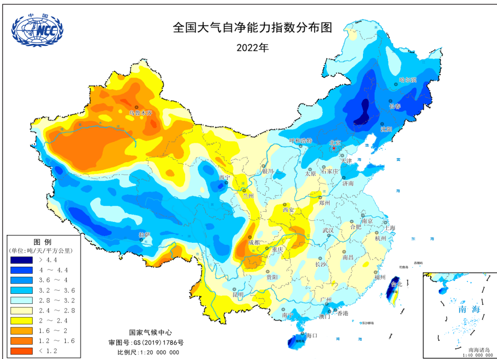
图61 2022年全国大气自净能力指数分布图(单位:吨/天/平方公里)
