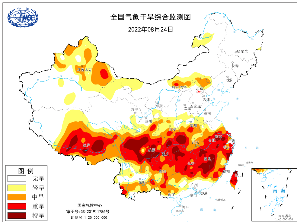
图42 2022年8月24日全国气象干旱综合监测图
