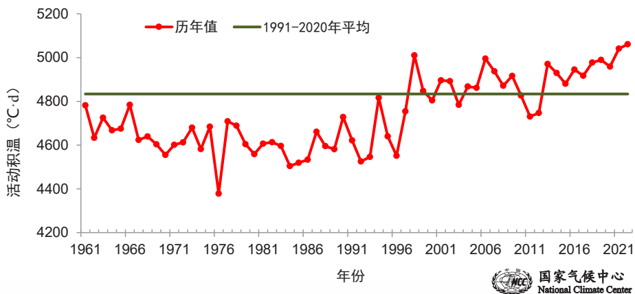
图8 1961-2022年全国平均 \geq 10^{\circ}\text{C} 活动积温历年变化 (单位: ^{\circ}\text{C}\cdot\text{d} )
