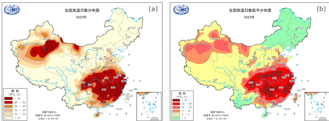
图7 2022年全国高温日数(a)及其距平(b)分布(单位:天)
