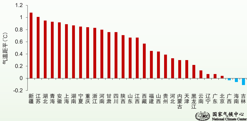
图3 2022年各省(区、市)平均气温距平 (单位: °C)
