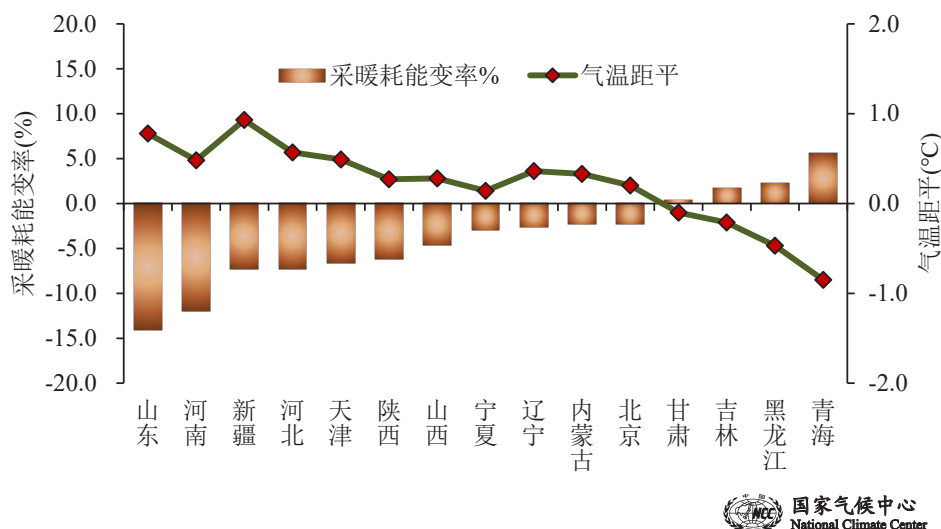
图56 2021/2022年冬季北方15省(区、市)采暖耗能变率(单位:%)和气温距平(单位:°C)
