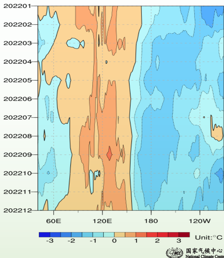
图25 2022年1-12月赤道印度洋和太平洋(5°S~5°N)海表温度距平时间-经度剖面(单位: ^{\circ}\text{C} )
