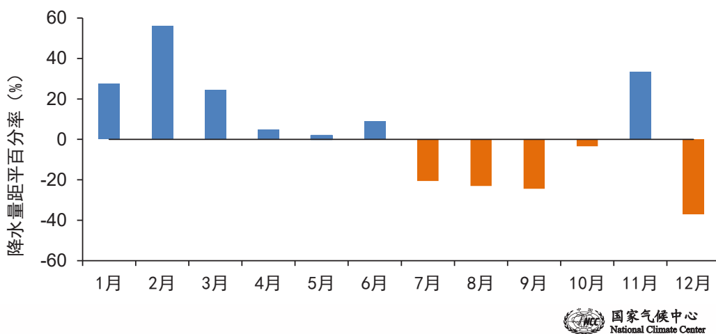
图14 2022年全国平均降水量距平百分率逐月变化(单位:%)
