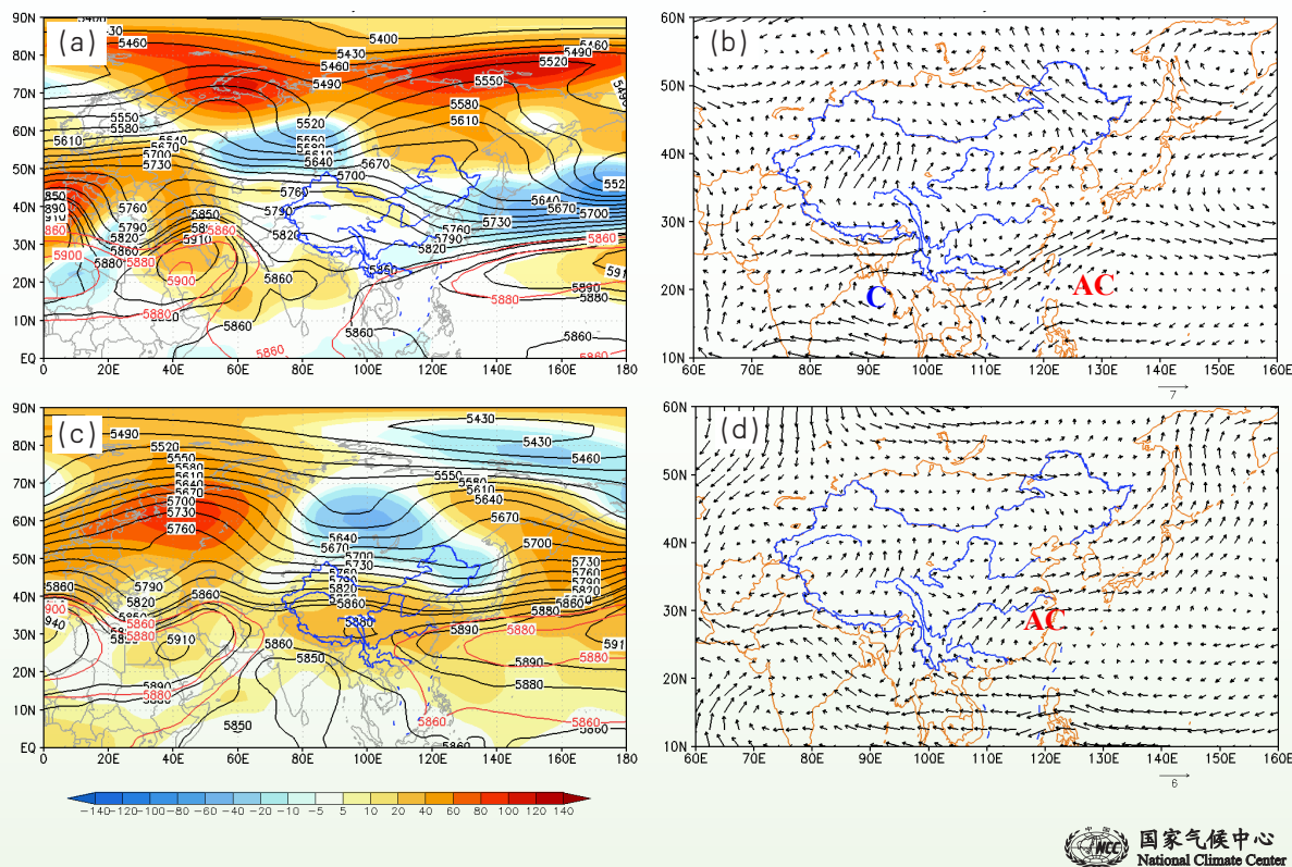
图36 2022年夏季6月上中旬 (a, b) 和6月下旬至8月 (c, d) 500hPa高度场 (a, c, 等值线单位: 位势米; 红色等值线表示常年的5880和5860位势米) 和距平场 (a, c, 阴影区单位: 位势米) 及850hPa风场距平 (b, d单位: 米/秒; AC: 反气旋; C: 气旋)
