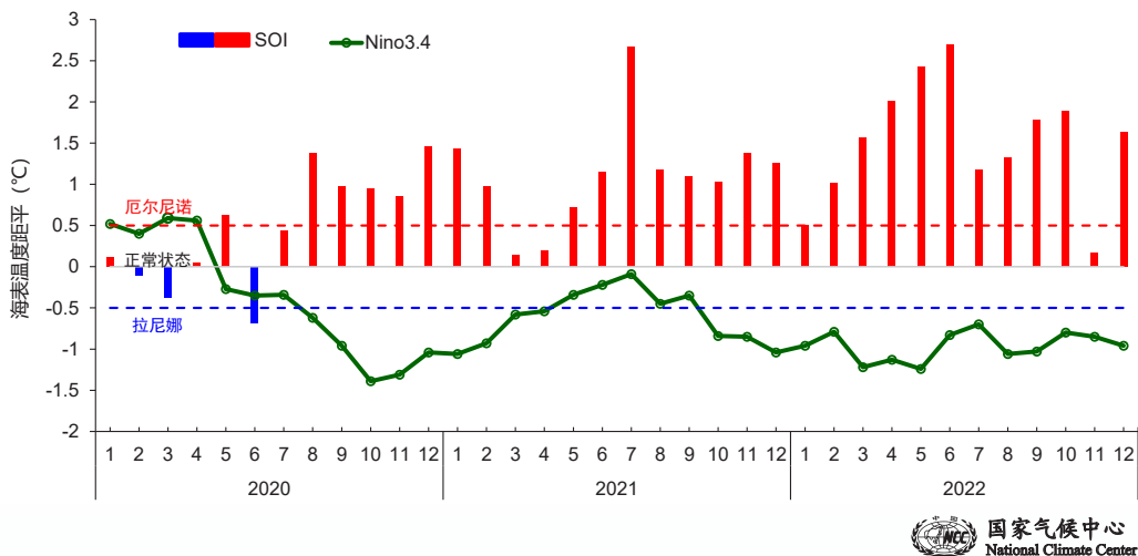
图26 2020年1月至2022年12月Niño 3.4指数 (单位: °C) 及南方涛动指数 (SOI) 逐月演变
