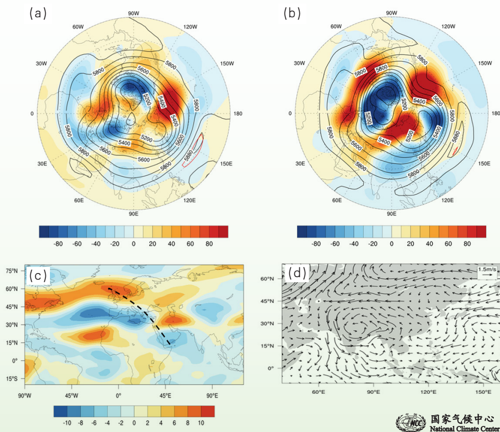
图30 2021年12月-2022年1月(a)及2022年2月(b)平均500hPa高度场(等值线)和距平场(阴影)(单位:gpm;红色等值线表示气候平均5880gpm)、冬季200hPa纬向风距平场(c)(单位:米/秒;黑色虚线表示波列)及冬季700hPa距平风场(d)(单位:米/秒)
