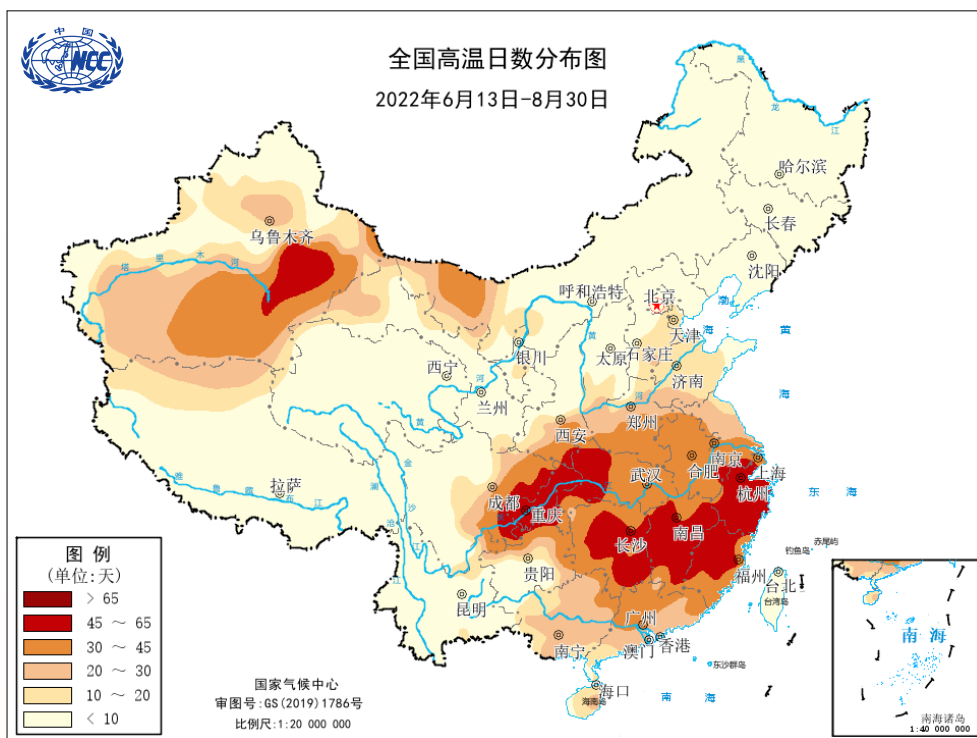
图48 2022年6月13日至8月30日全国高温日数分布(单位:天)
