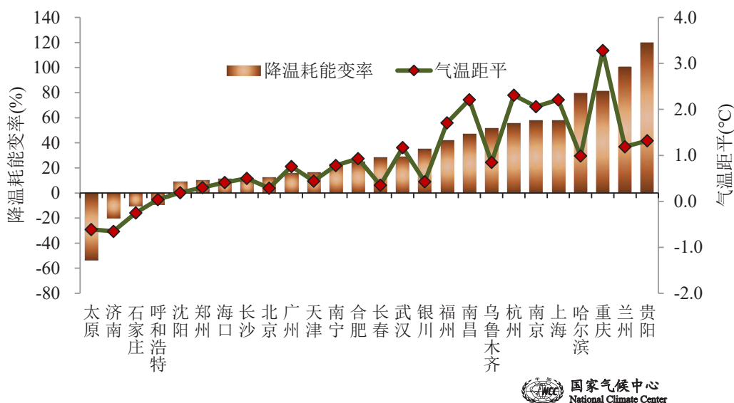
图57 2022年7月主要城市降温耗能变率(单位:%)和气温距平(单位:℃)
